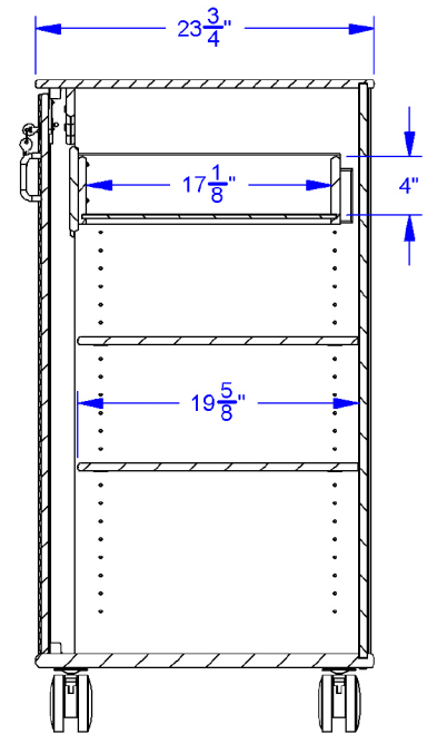
SECTION A-A
