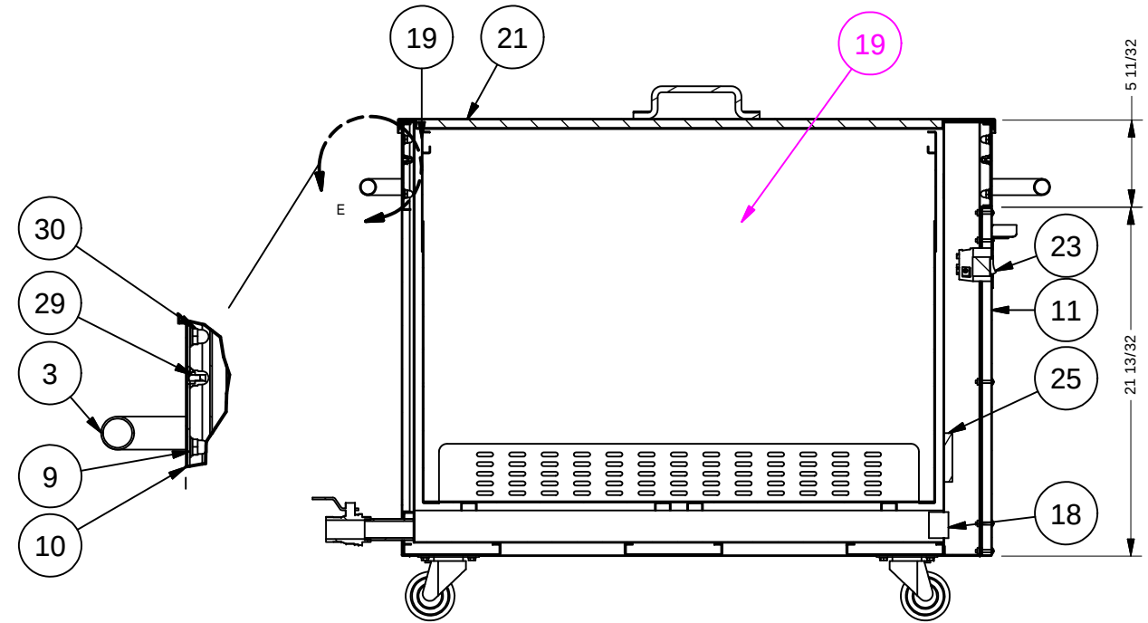
SECTION D-D
