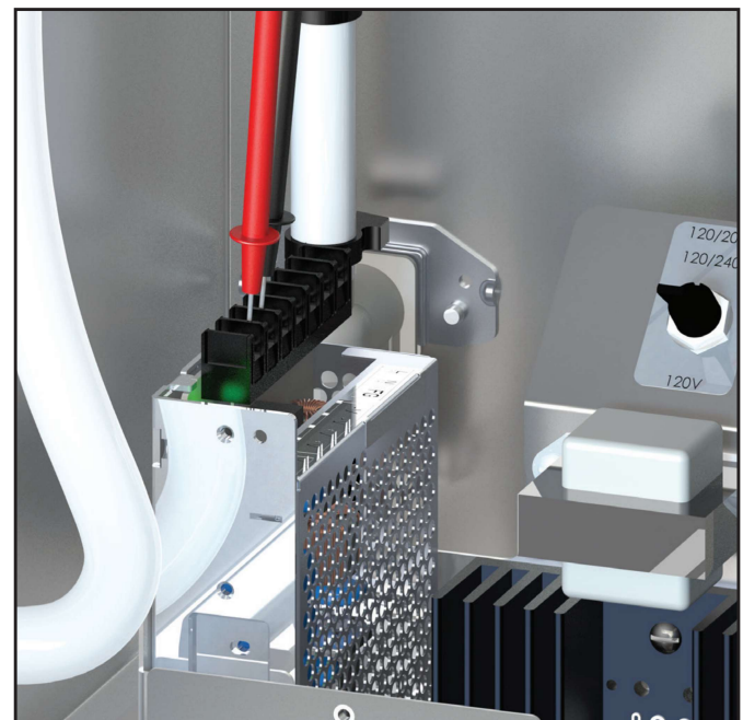
FIG. 23-3 TEST OUPUTS
