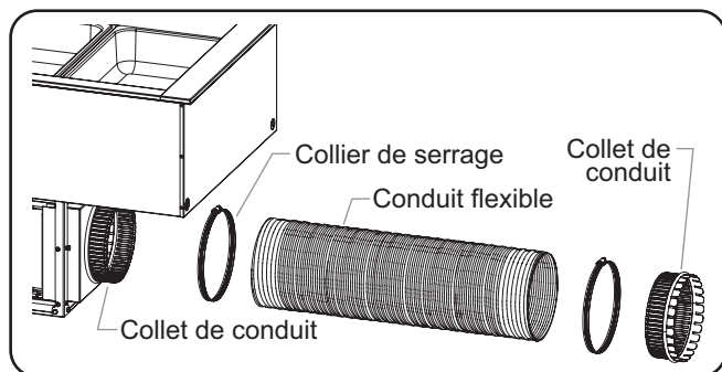
Installation du conduit flexible
