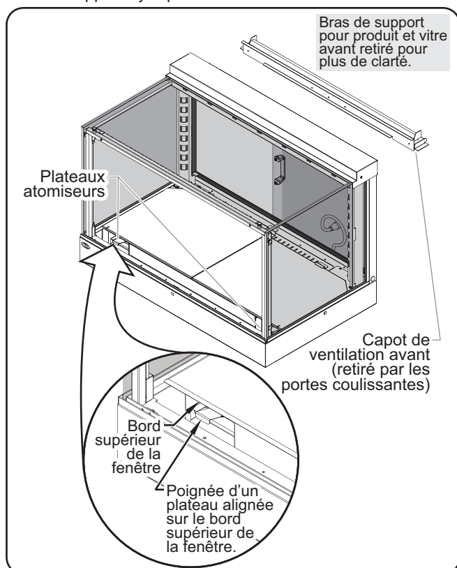
Vérification des plateaux atomiseurs (vue du IHDCH-45)
