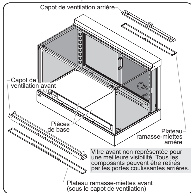
Retrait/installation des composants (vue du IHDC-45)
