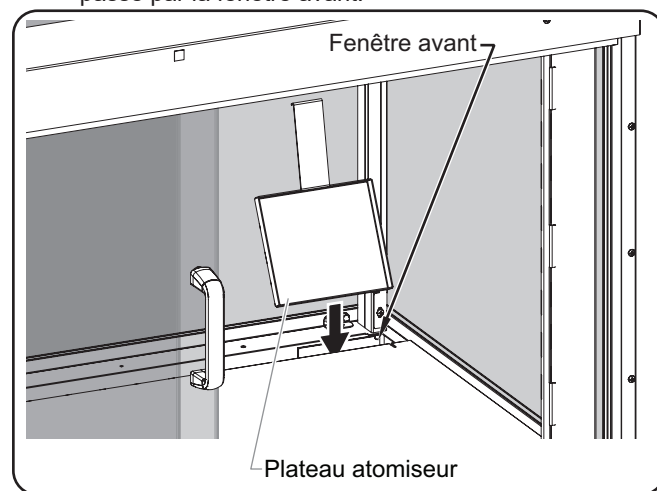
Retrait/installation des plateaux atomiseurs (vue du IHDCH-45)
