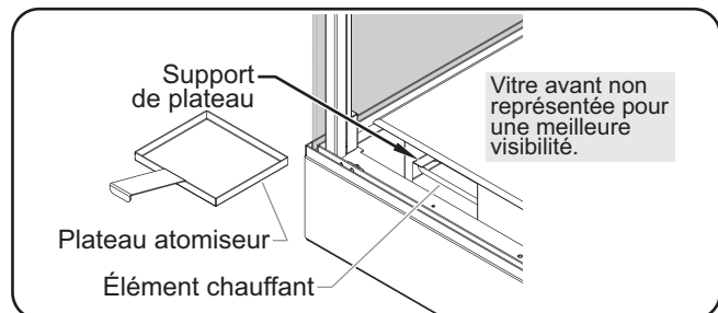
Disposition d'un plateau atomiseur (vue du IHDCH-45)
