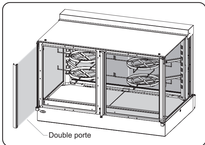
Double porte avant à fermeture automatique
