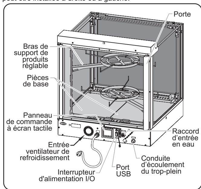
Vue arrière du modèle IHDCH-28
