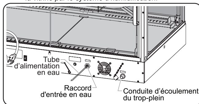
Raccordement de l'alimentation en eau (vue du IHDCH-45)
