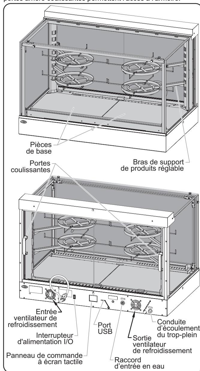
Vues avant et arrière du modèle IHDCH-45
