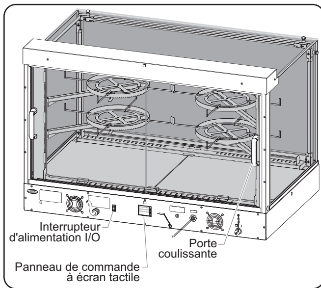
Commandes (vue du IHDCH-45)
