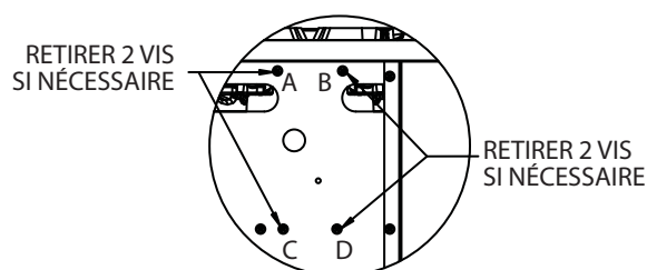
DÉTAIL II POUR CUISENIÈRE DE 60 PO AVEC FOUR STANDARD
